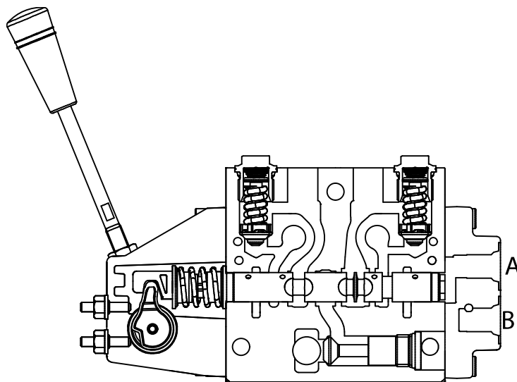
PVH actuation module
