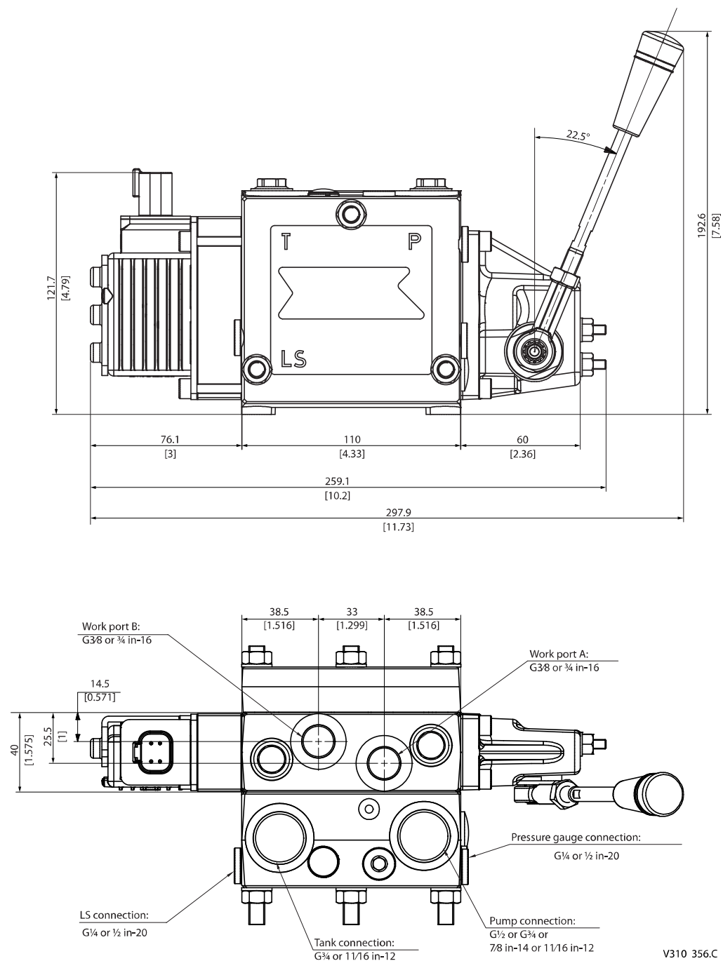
PVG 16 dimensions
